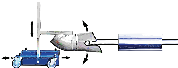
Positionierung des Trichters bei geradem Endrohr
